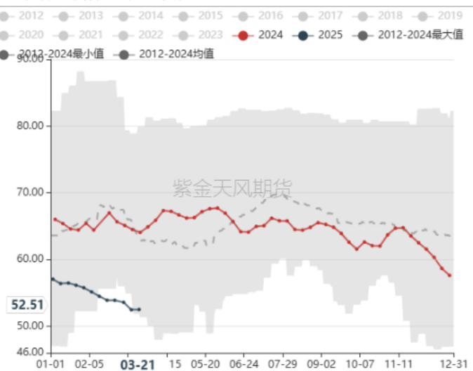
水泥熟料：库容比：中国（周）
