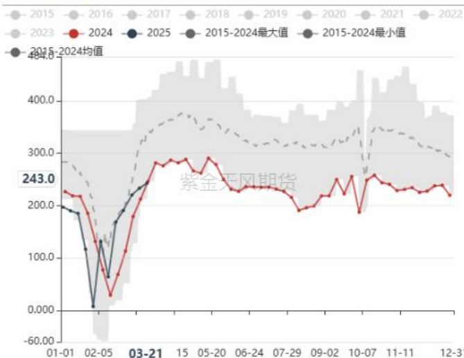
螺纹钢表观需求量：季节图 (万吨)
