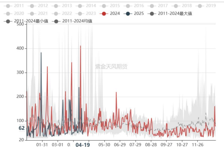
【SI】AQI指数:内蒙古:包头市
