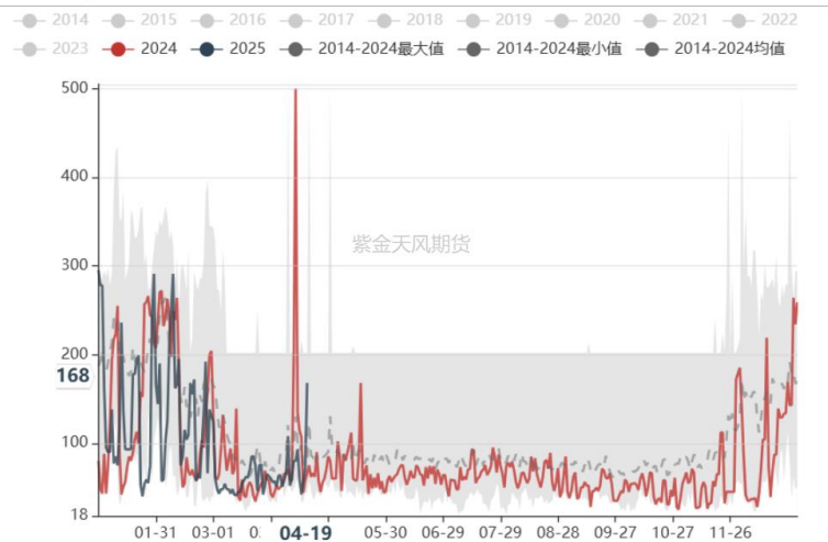
【SI】AQI指数:新疆:石河子市
