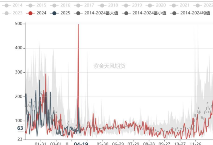
【SI】AQI指数:新疆:乌鲁木齐市
