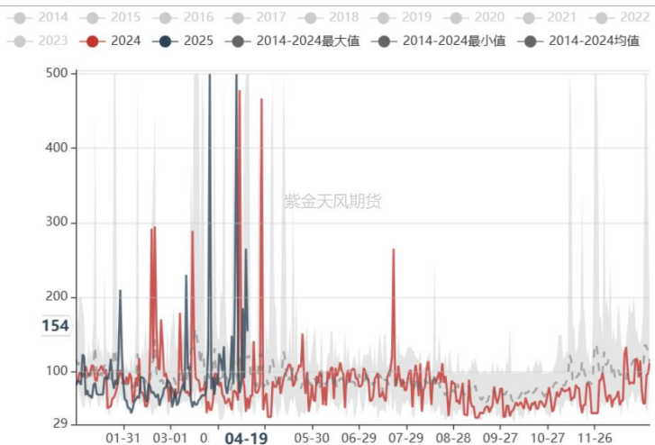
【SI】AQI指数:甘肃:兰州市
