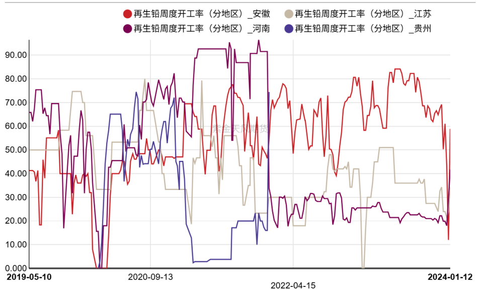
【PB】再生铅厂周度开工率-分地区
