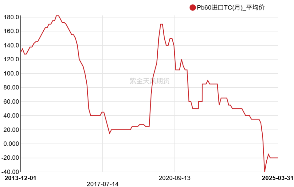
【PB】进口铅精矿月度TC（美元/干吨）
